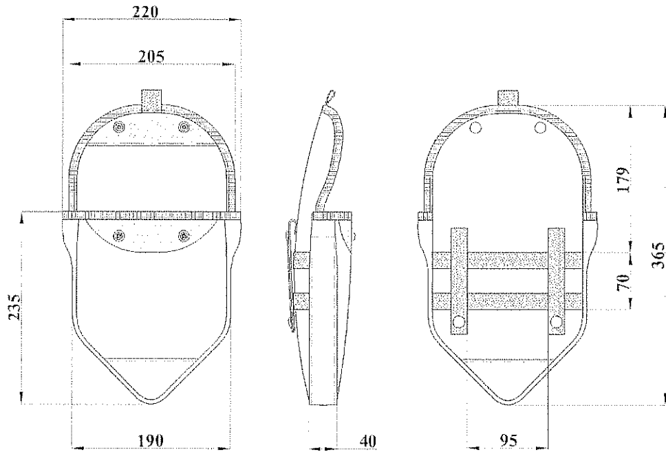
ФУТРОЛА ЗА АШОВЧИЊ
