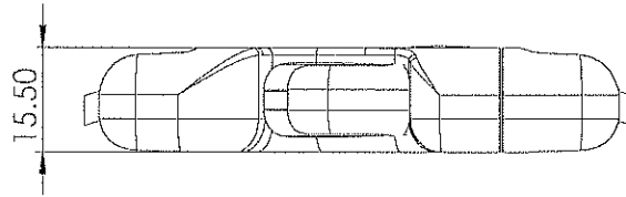
Слика 1 - Изглед и димензије бравице за опасач
