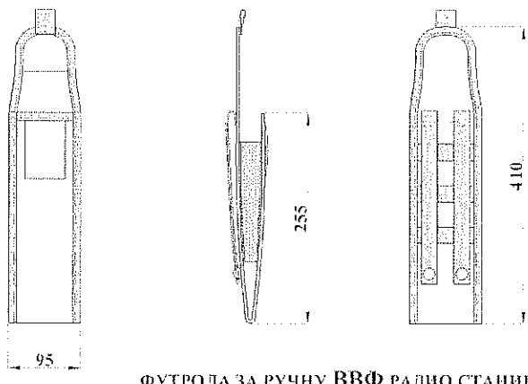
ФУТРОЛА ЗА РУЧНУ ВВФ РАДИО СТАНИЦУ
