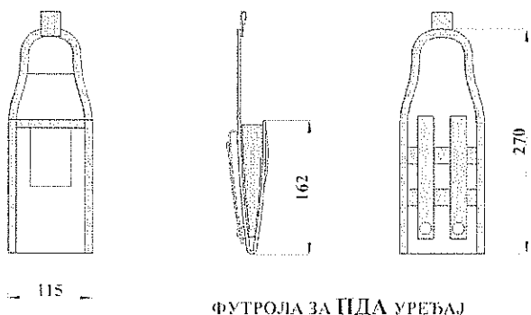
ФУТРОЛА ЗА ПДА УРЕЂАЈ
