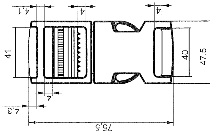
Слика 10. Изглед и димензије бравице за гуртну ширине 4 см
